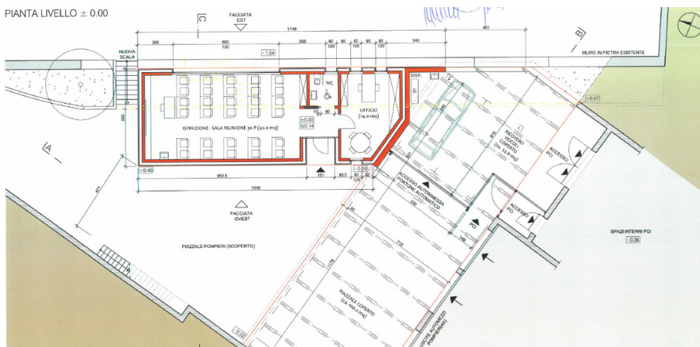
PIANTA LIVELLO ± 0.00
